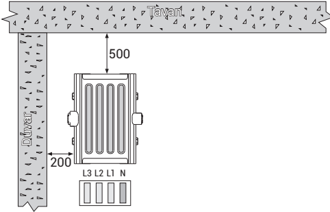
Şekil 2 - Dikey Pozisyon
